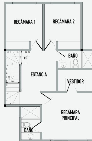
2DO NIVEL
